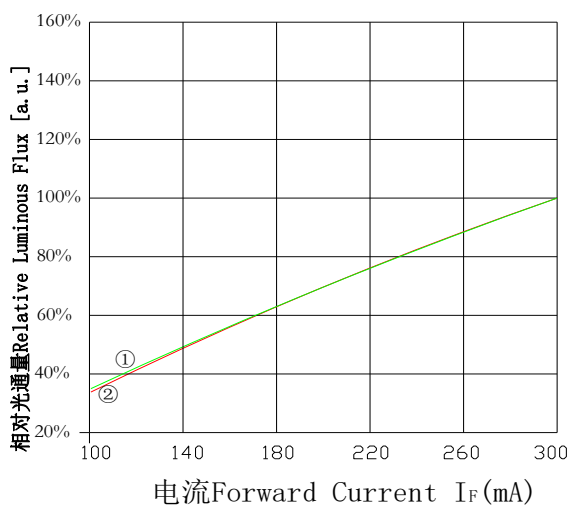
Forward Current vs.Relative Luminous Flux 正向电流与相对光通量曲线图
