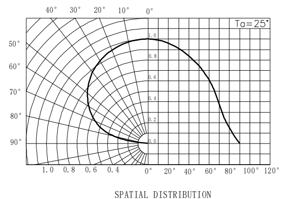
Radiation diagram 辐射图特性曲线
