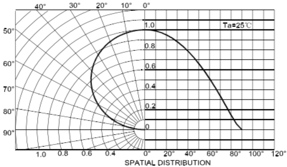
Radiation diagram 辐射图特性曲线
