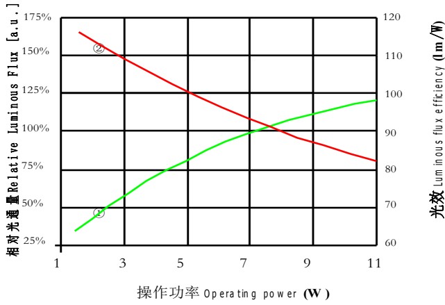
① ———— 操作功率对应相对光通量 ② ———— 操作功率对应光效
