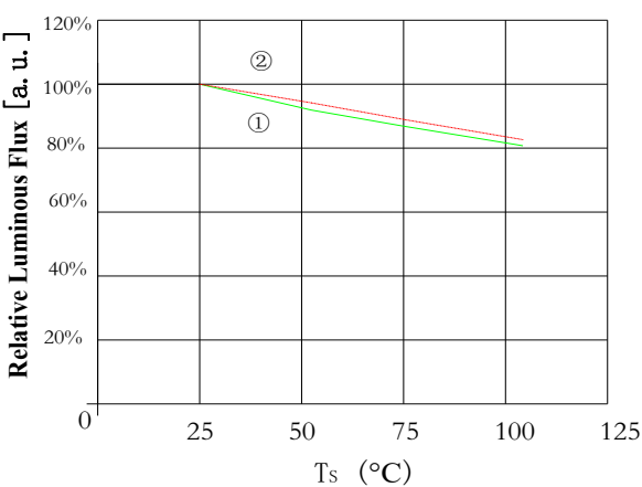
Case Temperature vs.Relative Luminous Flux 结点温度与相对流明曲线图 I_F=300\text{mA}
