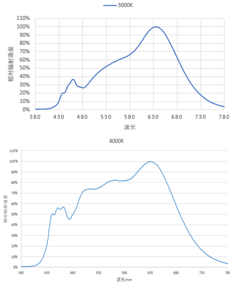
Relative spectral emission 相对光谱分布特性曲线
