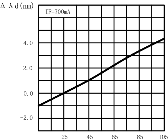
温度-波长漂移曲线
