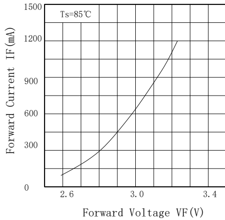
电流-正向电压曲线
