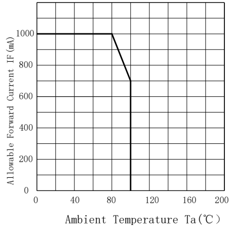
温度-正向电流曲线
