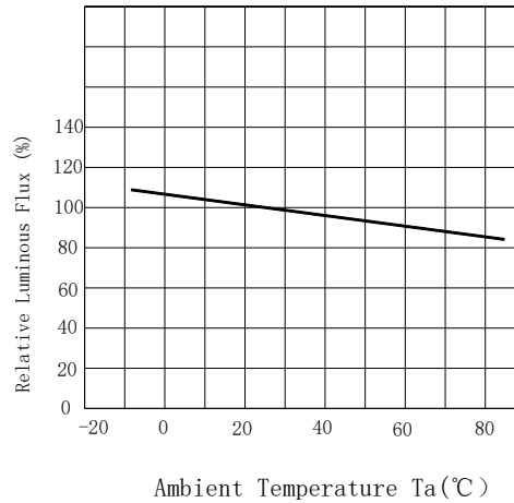
环境温度-相对光强曲线
