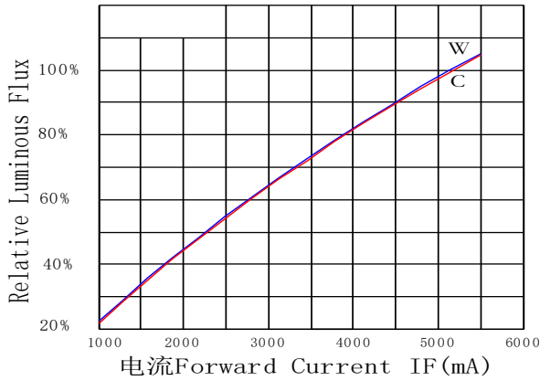
Relative Luminous Flux - IF 电流-相对光通量曲线(W&C)
