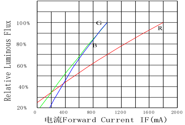
Relative Luminous Flux - IF 电流-相对光通量曲线 (R&G&B)
