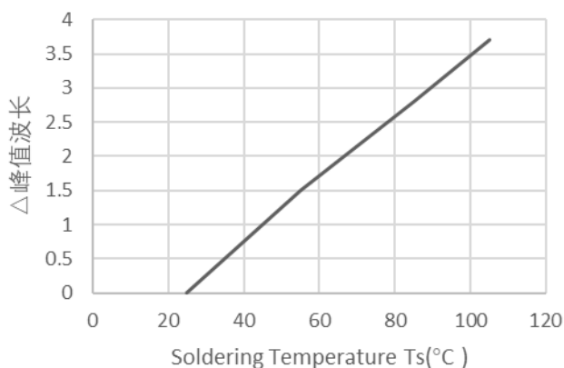
温度-峰值波长曲线
