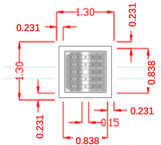
CSP Bottom View 背面图 单位: mm
