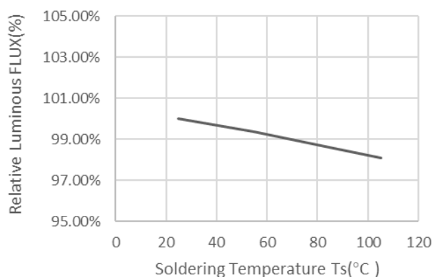
温度相对光通量曲线
