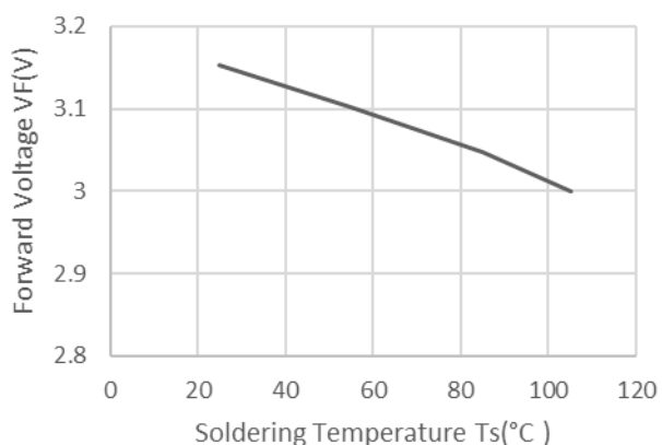
温度-正向电压曲线
