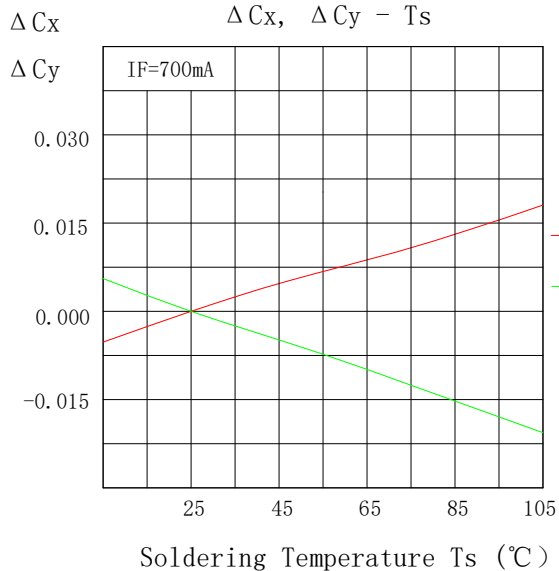
温度-色坐标漂移曲线
