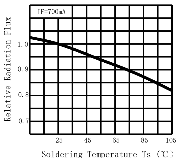
温度-相对辐射通量曲线
