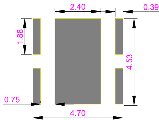
建议使用的钢网尺寸
