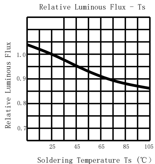
温度-相对光通量曲线
