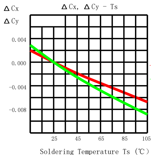
温度-色坐标漂移曲线
