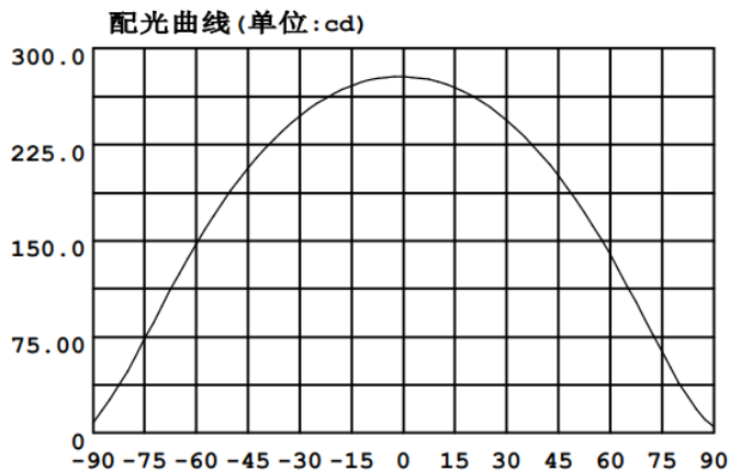
辐射模式
