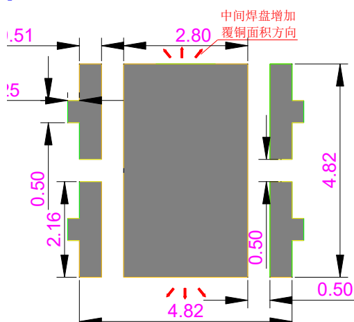
建议使用的焊盘尺寸
