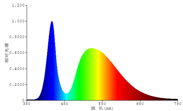
光谱曲线@ T_c=5700\text{K}
