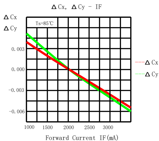
电流-色坐标漂移曲线
