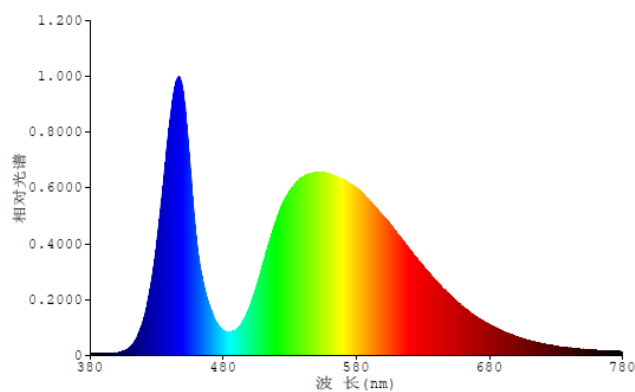
光谱曲线@ T_c=5700\text{K}
