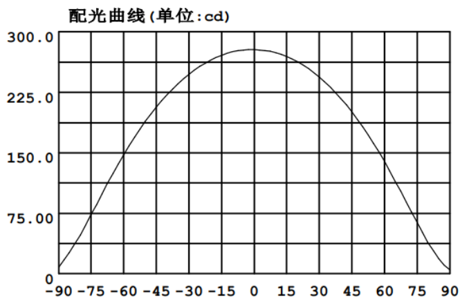
辐射模式
