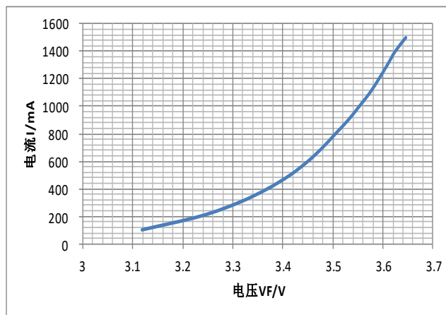
Fig.2- 伏安特性曲线
