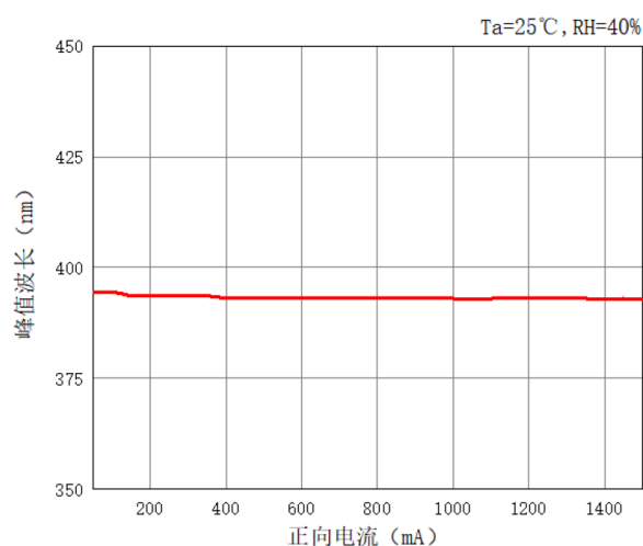
Fig.4- 峰值波长与正向电流图
