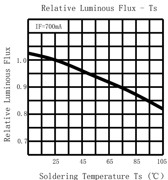
温度-相对光通量曲线
