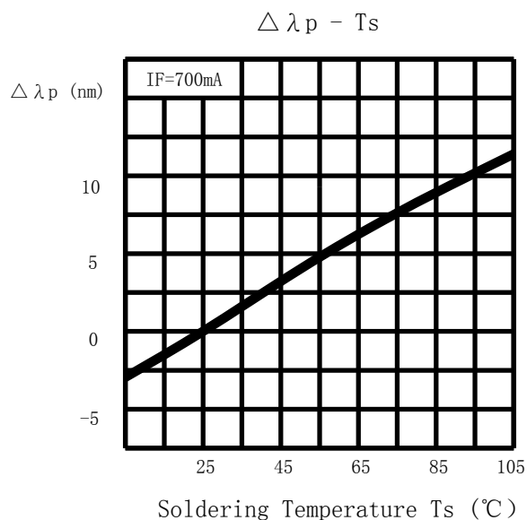
温度-波长漂移曲线
