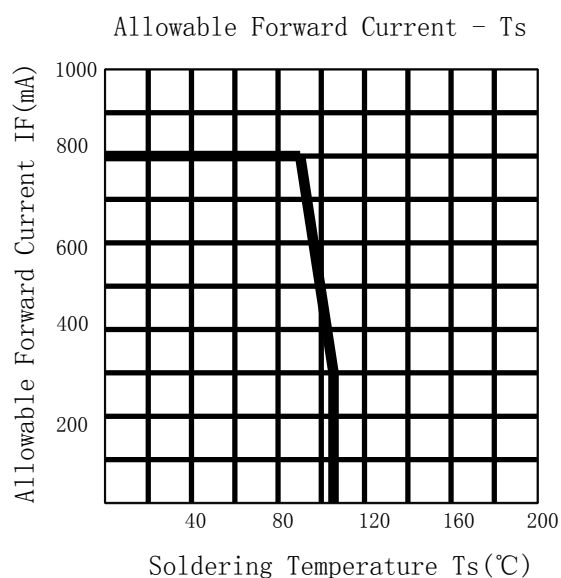
温度-最大允许操作电流
