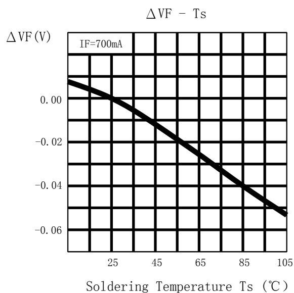
温度-正向电压曲线
