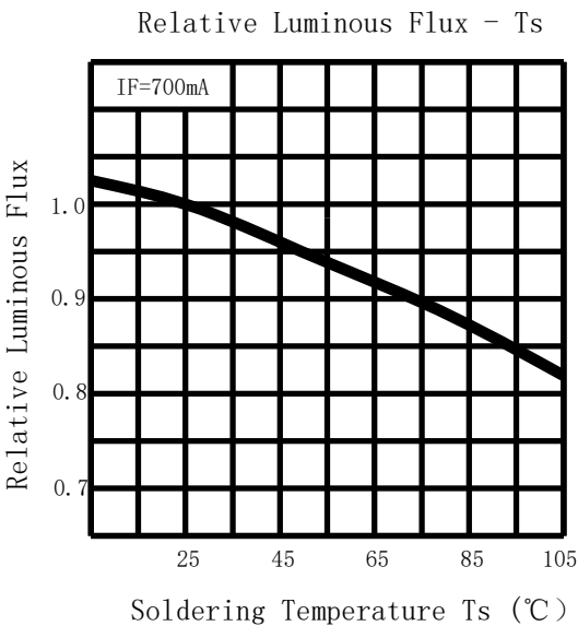
温度-相对光通量曲线
