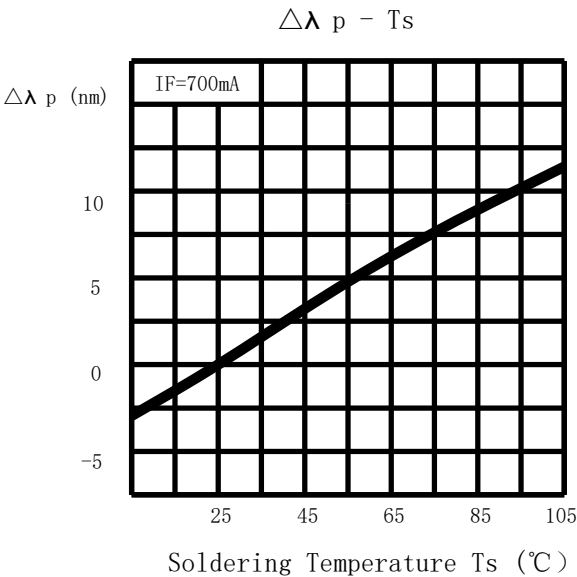
温度-波长漂移曲线
