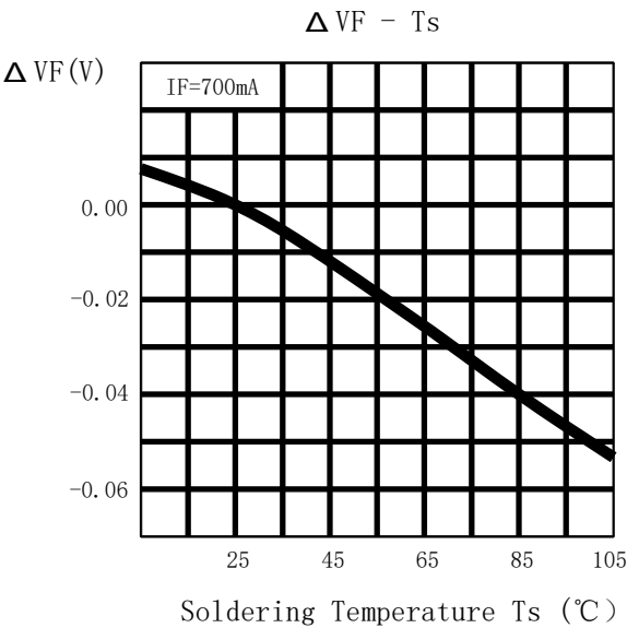
温度-正向电压曲线
