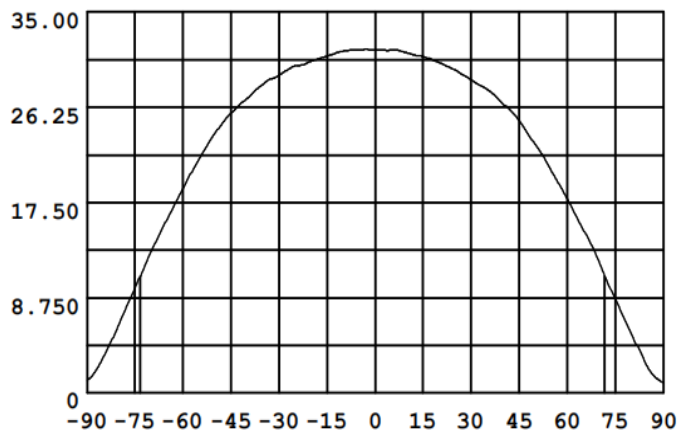
配光曲线 (单位: cd)
