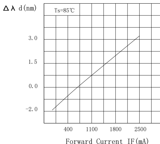
电流-波长漂移曲线
