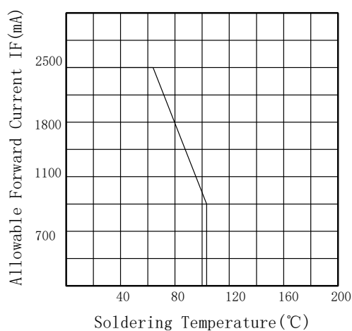
温度-最大允许操作电流
