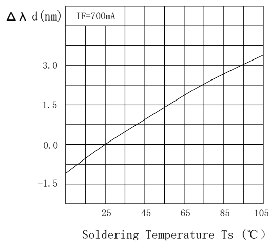
温度-波长漂移曲线
